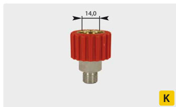
M22 h : rosca m. máx. 250 bar / 120 °C
