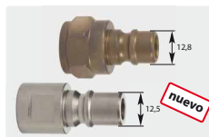
racor : rosca h. acero inox templado. máx. 350 bar / 100 °C
