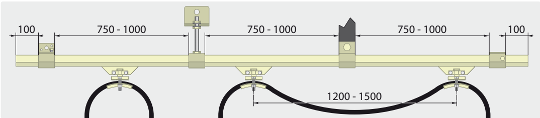
perfil de carriles guía
