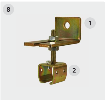
abrazadera ajustable + soporte pared
